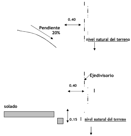
MODIFICACIÓN A LA TOPOGRAFÍA DEL TERRENO (FIG 3)
