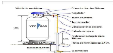
b.2) Sistema Garrafón de Gas Propano a Grael
